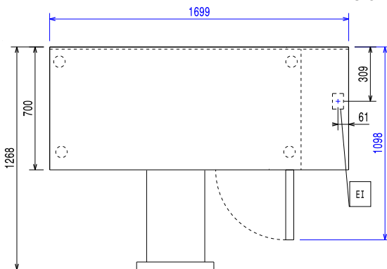
Felülnézet
